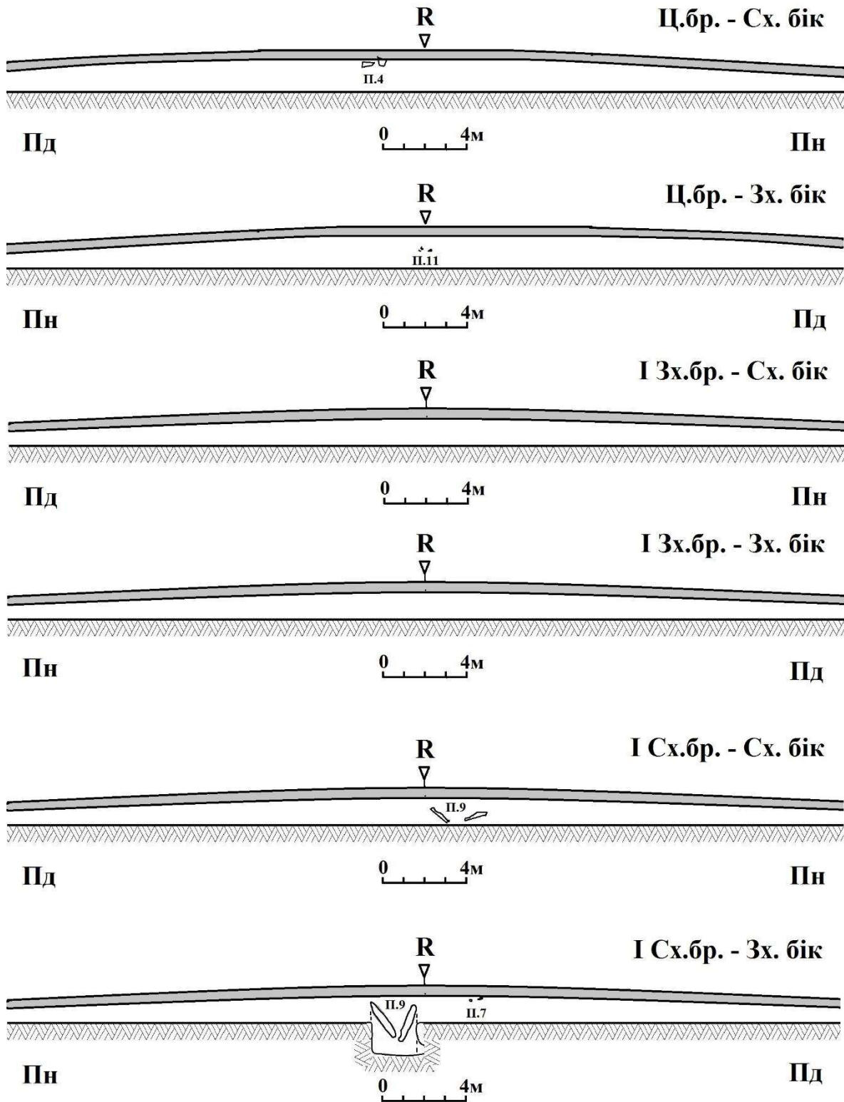
Рис. 3. Стратиграфічні розрізи.
